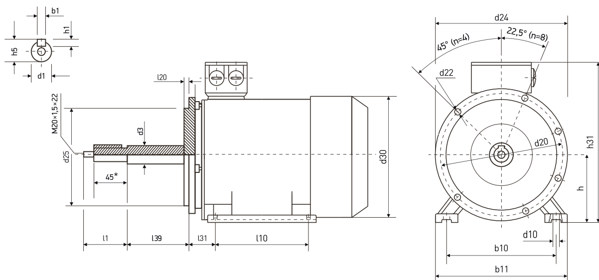
АИР 132, 160, 180, 200 Ж
