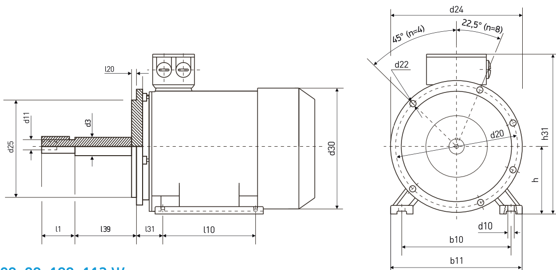
АИР 80, 90, 100, 112 Ж
